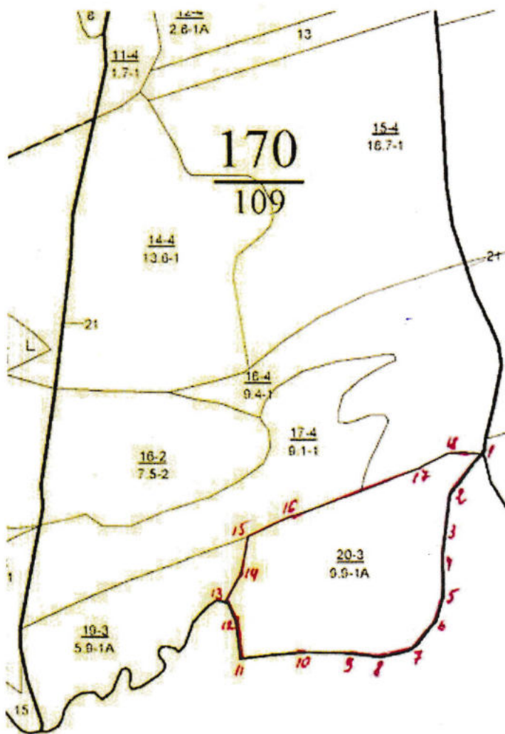
Румбы и длины линий
