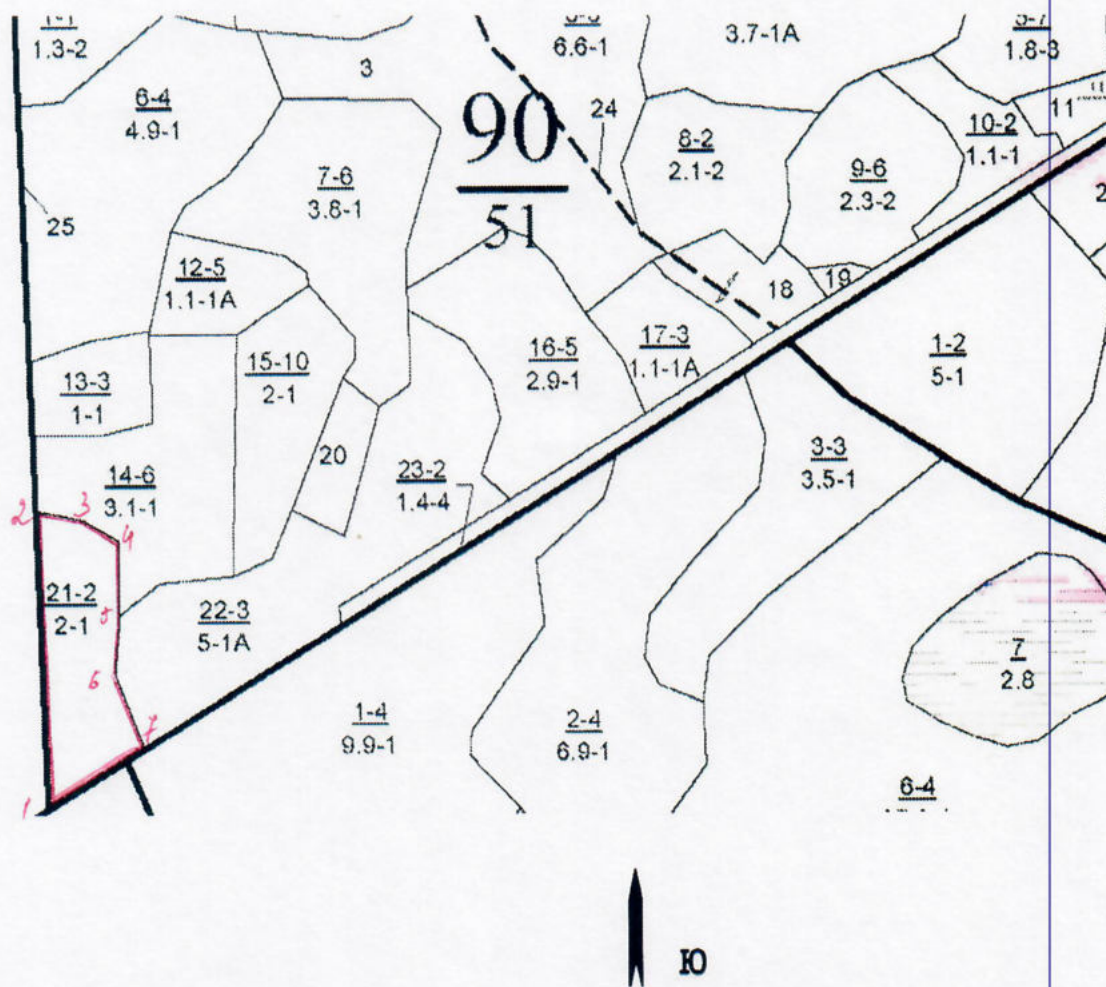
Румбы и длины линий
