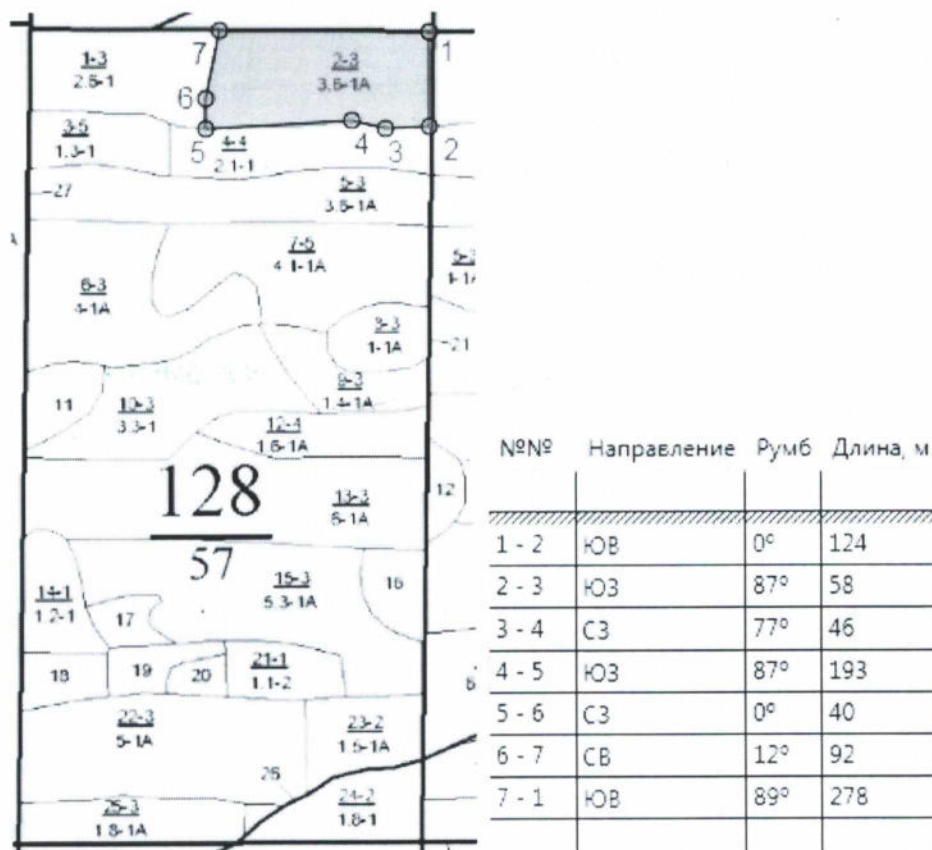
Общая схема участка и его привязки Румбы и длины линий
