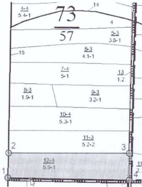
Общая схема участка и его привязки Румбы и длины линий
